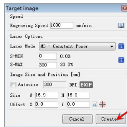
Nastavení velikosti obrázku a parametrů laseru
