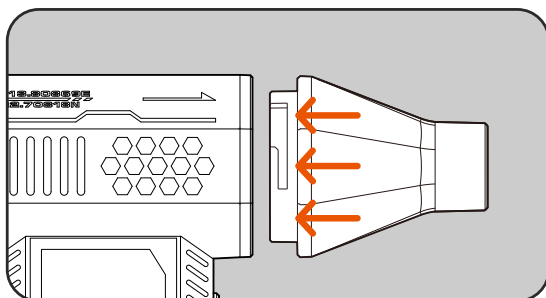
C: Aliniați clema duzei noi cu canelura aparatului și introduceți-o vertical la locul ei.
